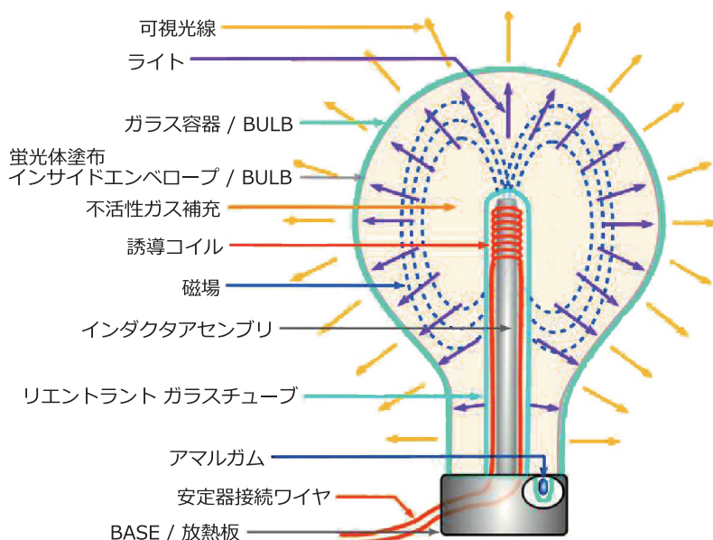
【低周波無電極ランプ (135Khz) 構造】
